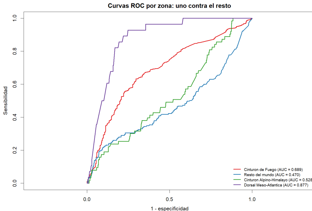
Figura 9. Curvas ROC por zona bajo comparación uno contra el resto.
